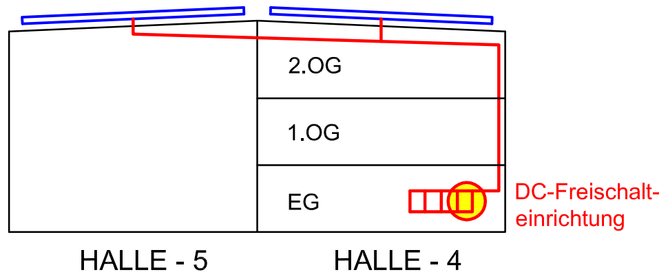
Schnitt: "A"
